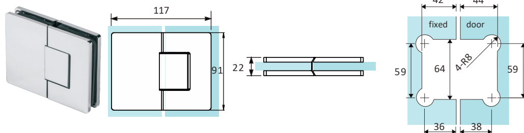
ガラス加工図
